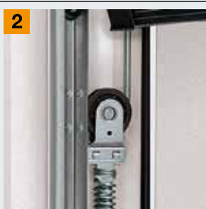
Система с разтегателни пружини
